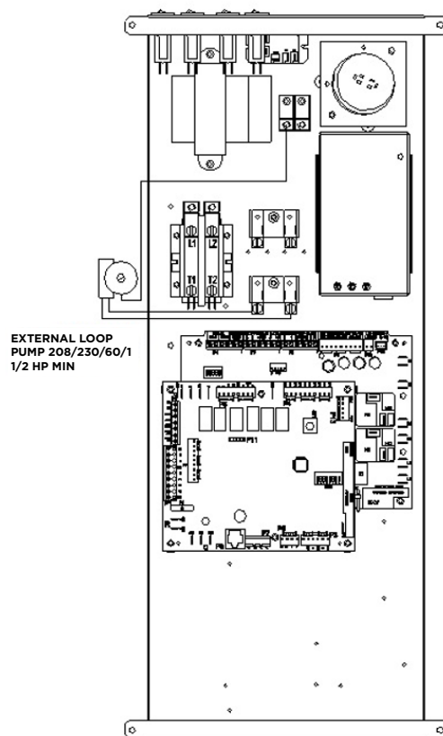
Figure 5 : Câblage de la pompe source 208-230/60/1
