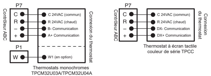
Figure 22 : Câblage du thermostat (signaux de communication)
