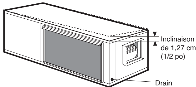
Figure 6 : Hauteur de l'unité pour le drain
