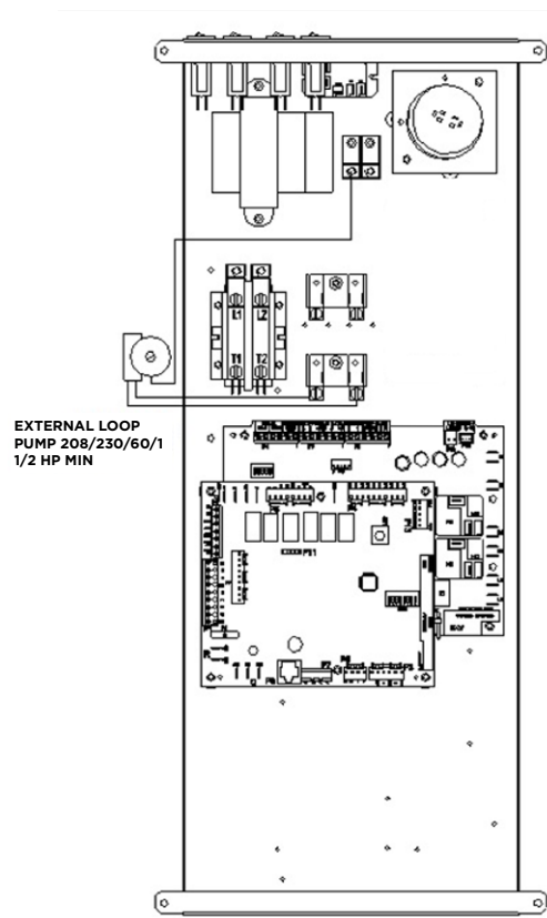
Figure 5 : Câblage de la pompe de source 208-230/60/1
