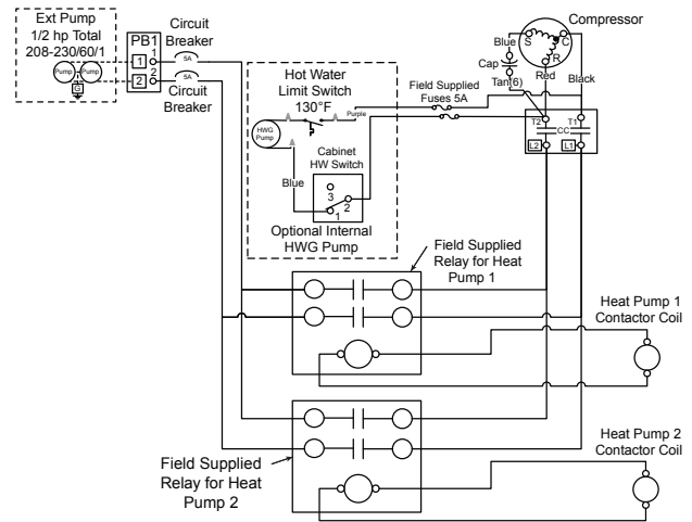
Figure 2a : Câblage primaire/secondaire avec commande de base Aurora (pas de carte AXB)
